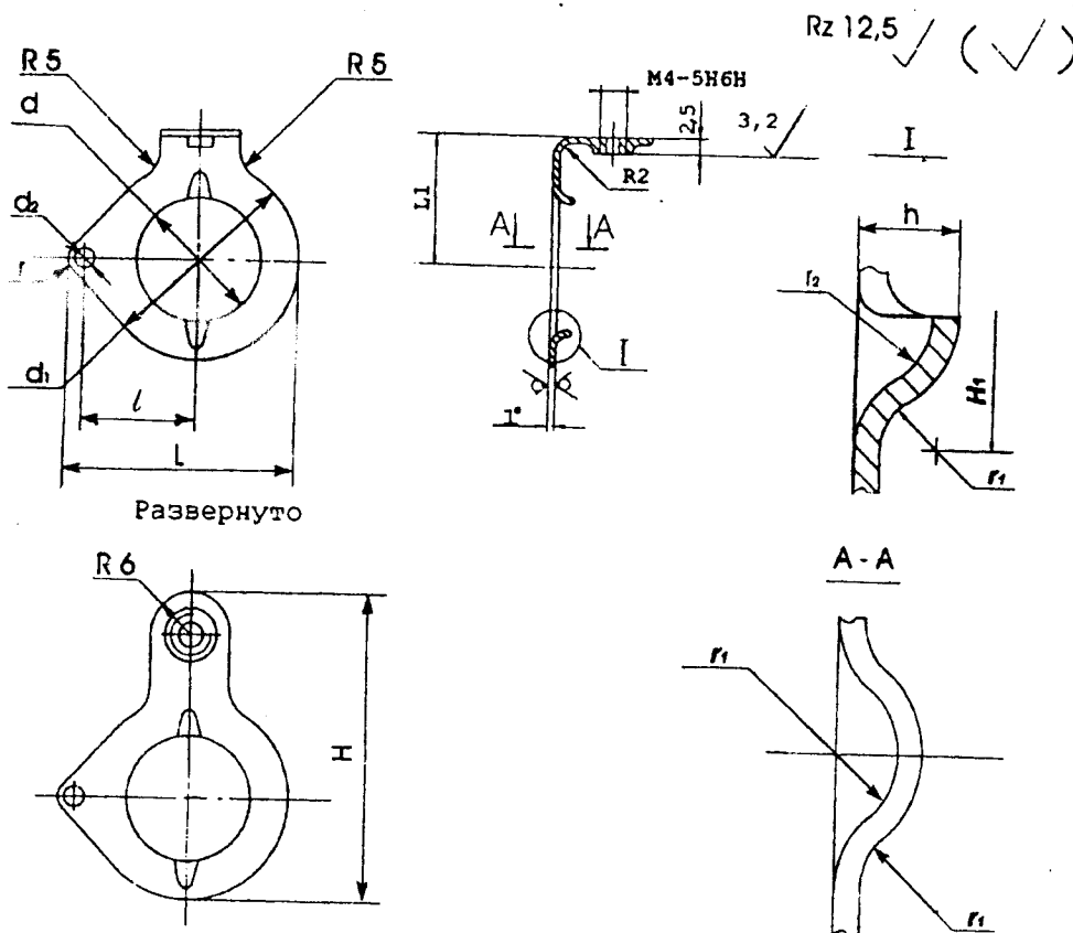
Размеры, мм
