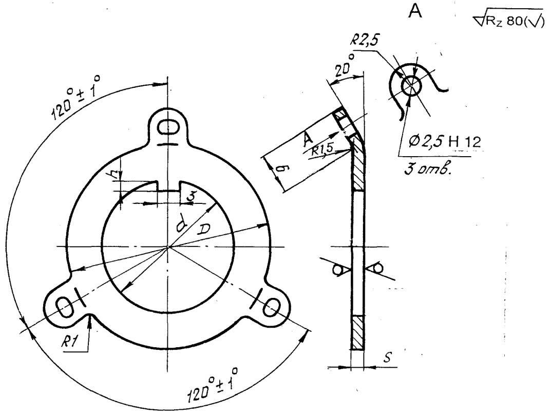
Размеры, мм
