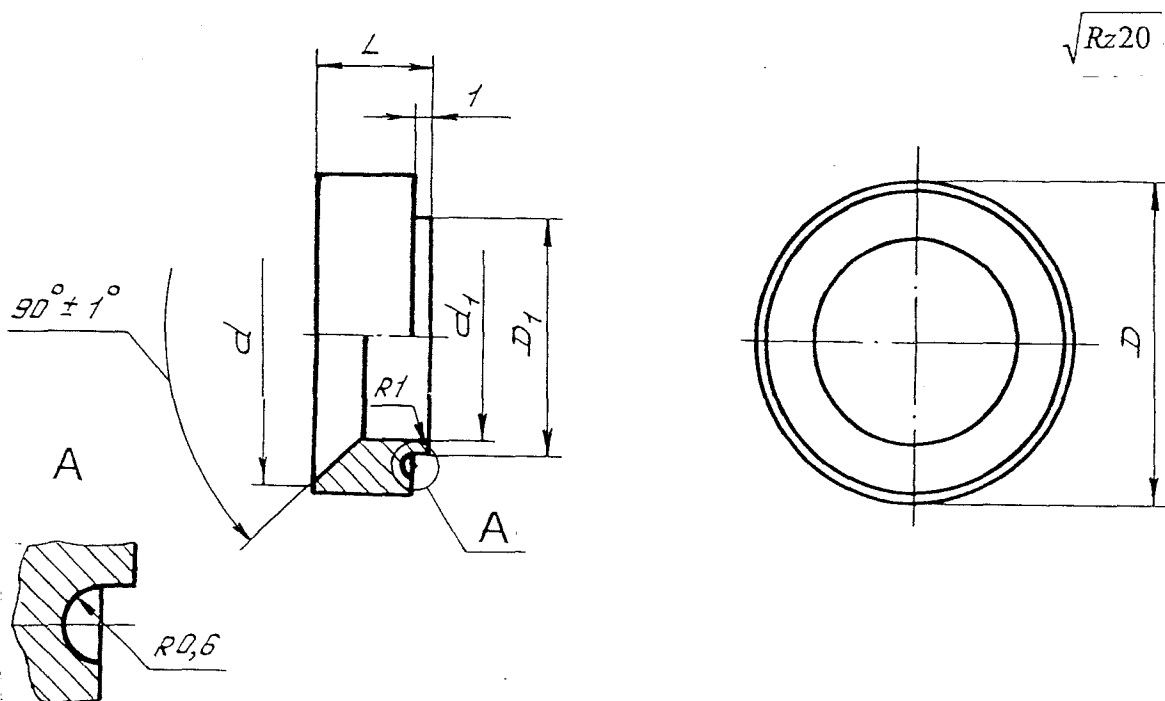
Размеры, мм
