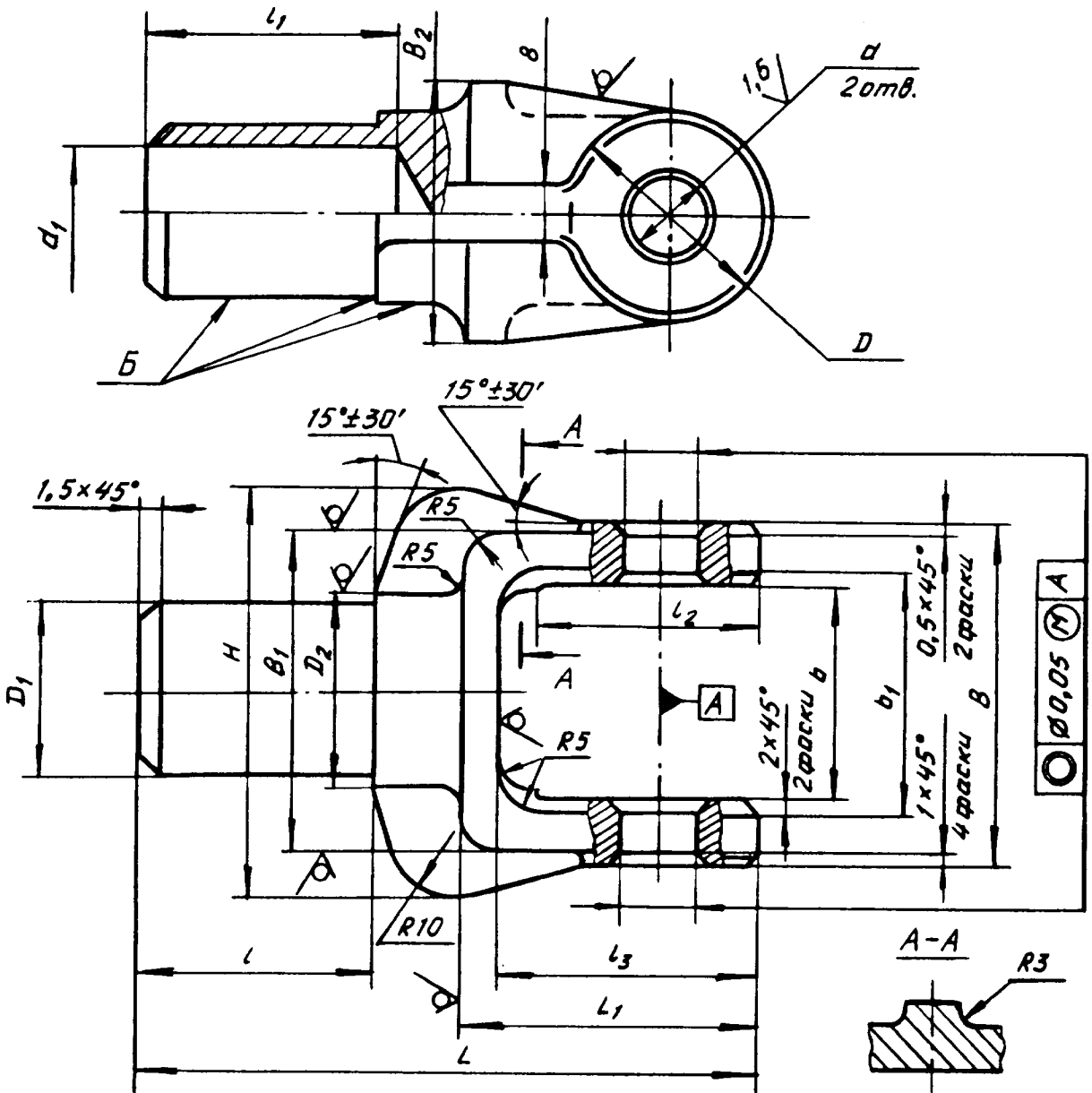
Размеры, мм
