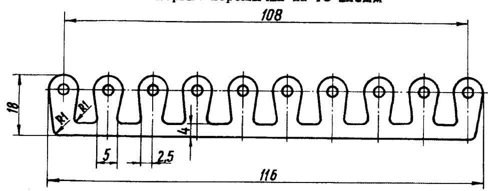
Развертка перемычки на 10 клемм
