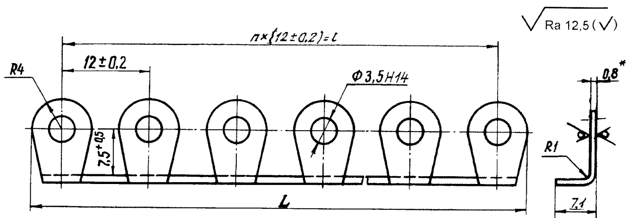
Развертка перемычки на 10 клемм
