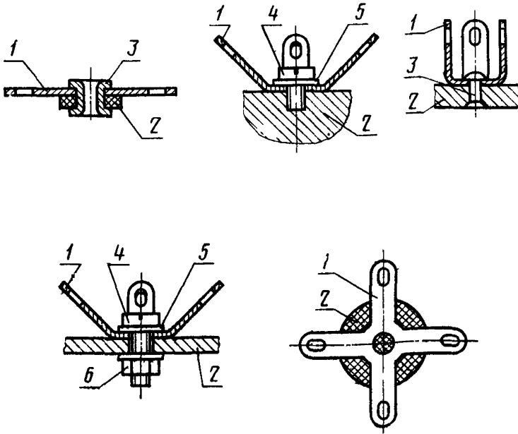
1—лепесток; 2—основание; 3—заклепка; 4—винт; 5—шайба; 6—гайка.
